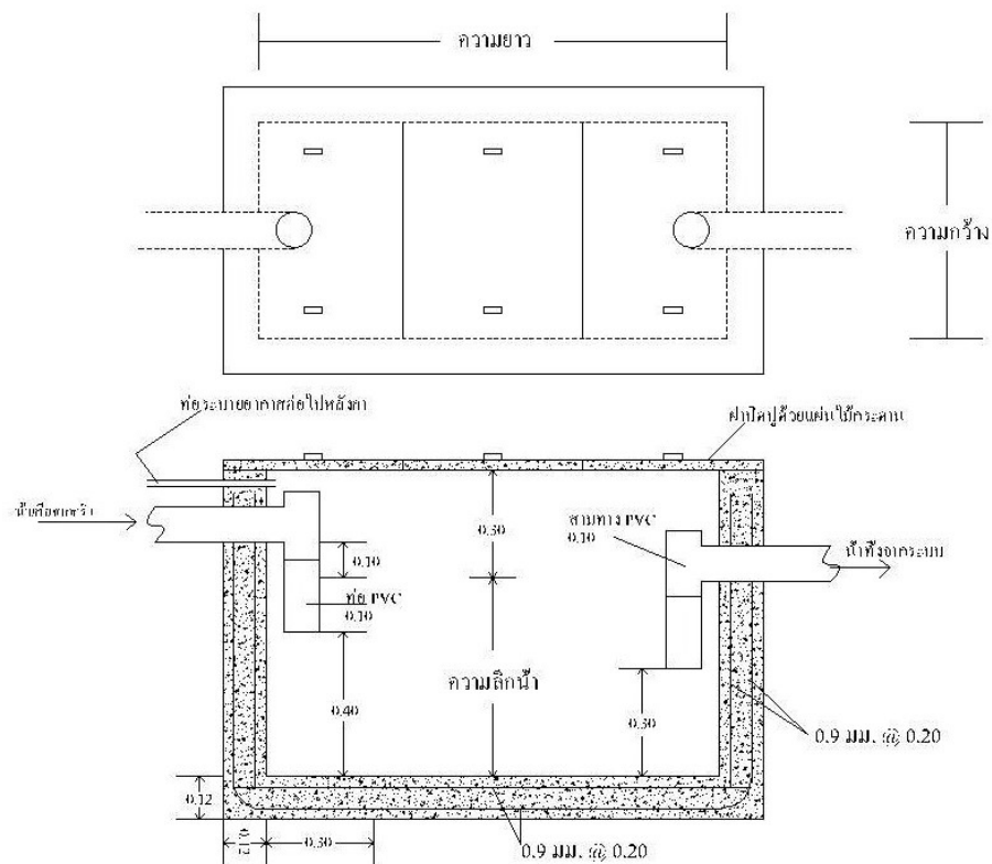
บ่อพักน้ำแบบสร้างในที่สำหรับอาคารขนาดใหญ่
