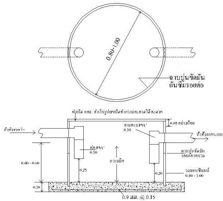
บ่อพักน้ำแบบวงขอบซีเมนต์สำหรับบ้านพักอาศัย
